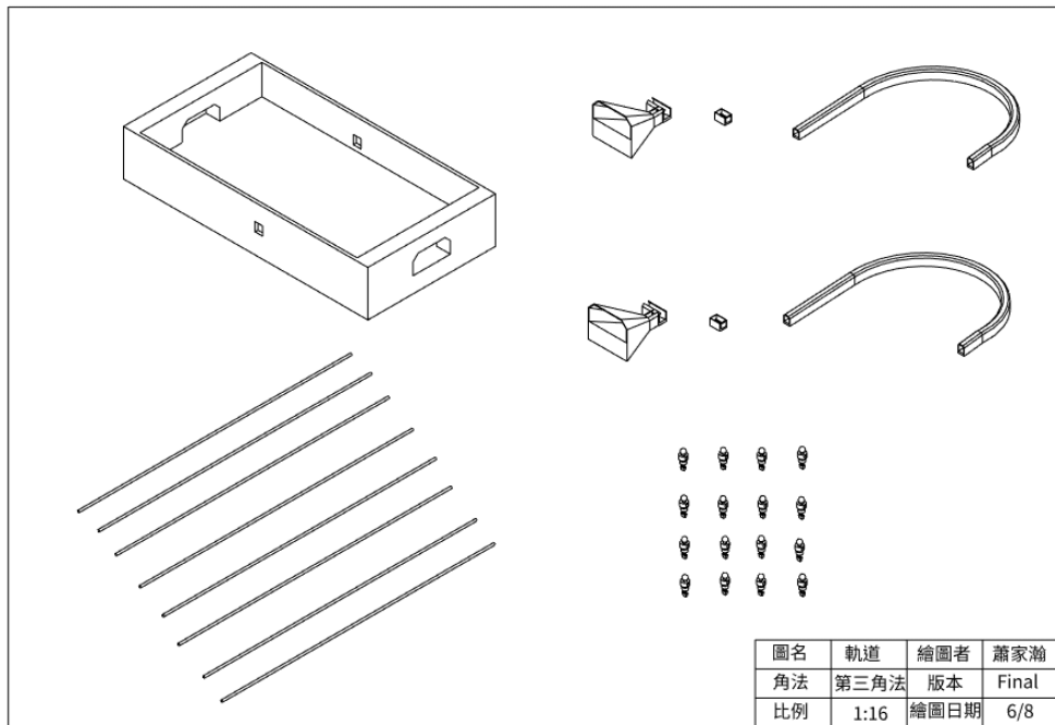
組合圖 BOM
